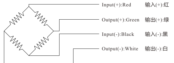
Wiring Diagram/接线图
