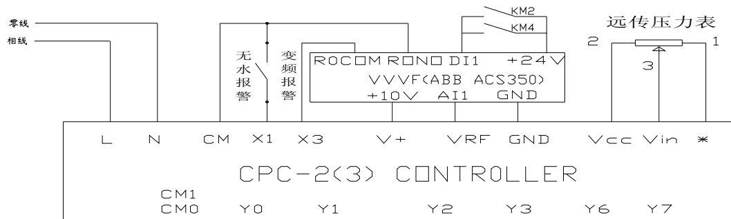
图五 ABB ACS350变频器与控制器接线图
