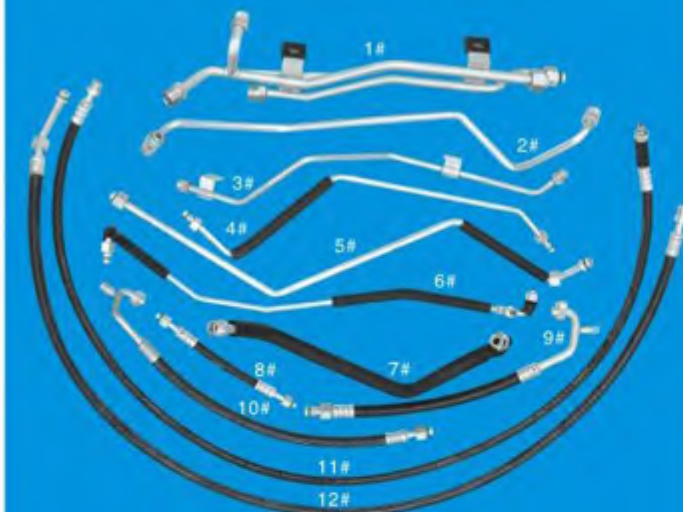
五菱之光管路总成 Wuling Zhiguang pipeline assembly
