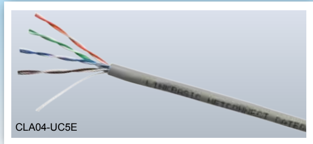
Cat 5E UTP solid cable RAL 7035
