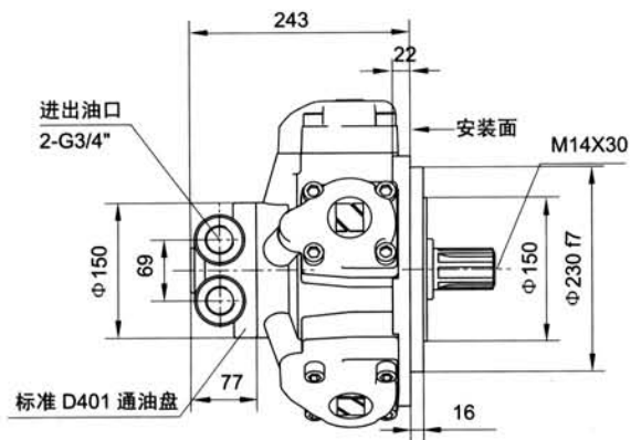
标准外花键 JMDG6-**A
