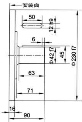
标准平键 JMDG6-**B
