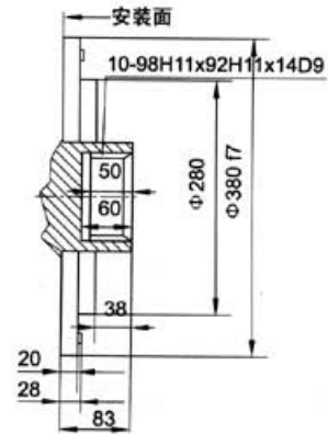
标准内花键 JMDG31-***I
