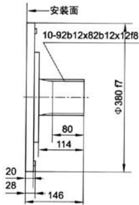
标准外花键 JMDG31-***A
