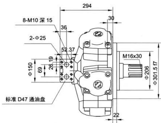
标准外花键 JMDG16-**A
