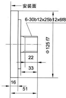
标准外花键 JMDG1-***A
