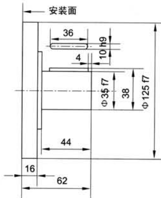
标准平键 JMDG1-***B
