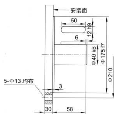
JMDG2-**S18
