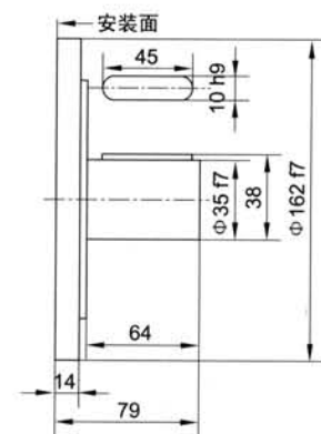
JMDG2-**B3
