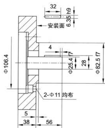
JMDG2-**B2
