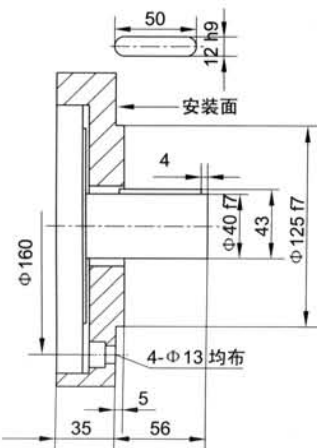
JMDG2-**B1
